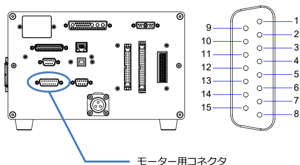
モーター用コネクタ
